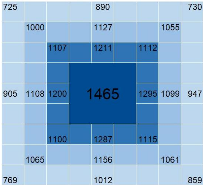
600W LM301H @ 15 cm Altura / 1,44 m 2
