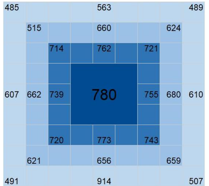
600W LM301H @ 60 cm Altura / 1,44 m 2
