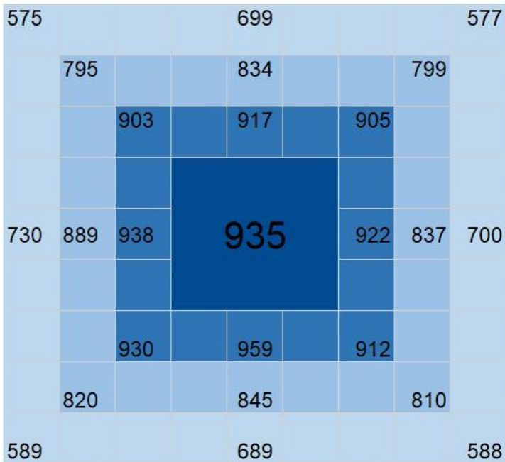
600W LM301H @ 45 cm Altura / 1,44 m 2
