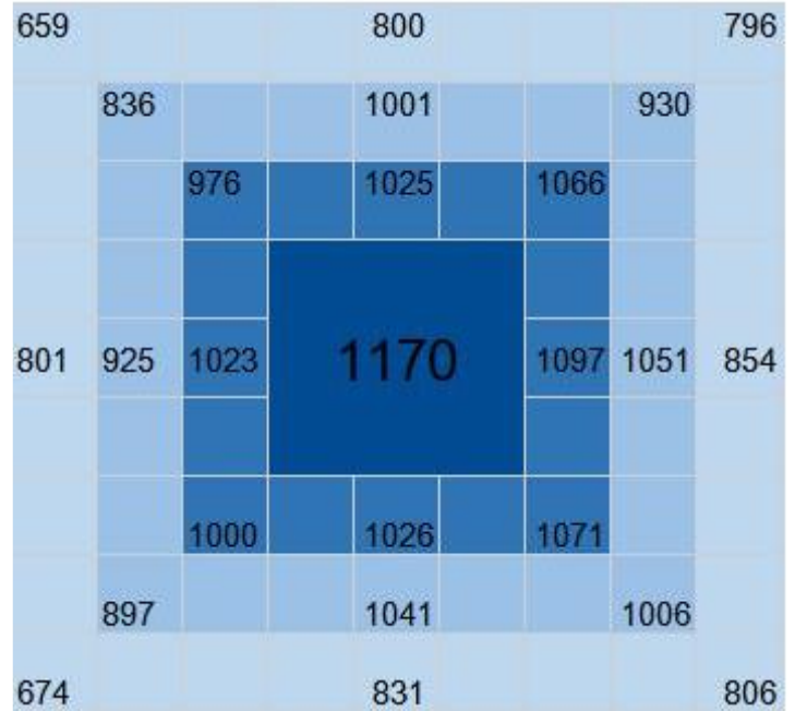
600W LM301H @ 30 cm Altura / 1,44 m 2
